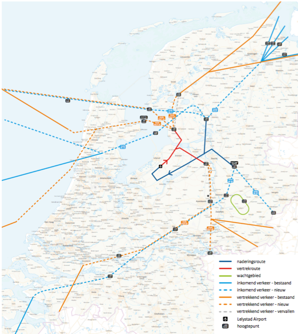
Figuur 2.3 Routestelsel voor uitgaand en inkomend verkeer bij starten en landen in noordoostelijke richting; ongeveer 40% van de tijd. Zie bijlage 1 voor uitsneden met leesbare hoogteaanwijzingen. (versie 7 februari 2018).
