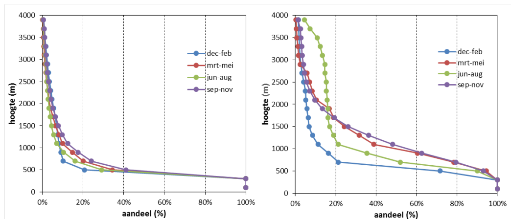
Figuur 3.5 Cumulatieve verdeling van dichtheidsklassen 10-40 \text{ ex/km}^3 (birdtam 5, 6, rechts) en >40 \text{ ex/km}^3 (Birdtam 7 en 8, rechts) over de kolom van 200-4.000 m hoogte; uitgedrukt als aandeel (%) van het absoluut uren dat de dichtheid cumulatief is vastgesteld (figuur 3.1 en 3.3).
