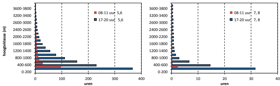
Figuur 3.9 Cumulatieve verdeling van dichtheidsklassen 10-40 ex/km 3 (Birdtam 5, 6) en >40 ex/km 3 (Birdtam 7, 8) over de kolom van 200-4.000 m hoogte voor 4 uren overdag en vier uren in de avond (donker); uitgedrukt in gemiddeld aantal uren per drie maanden..
