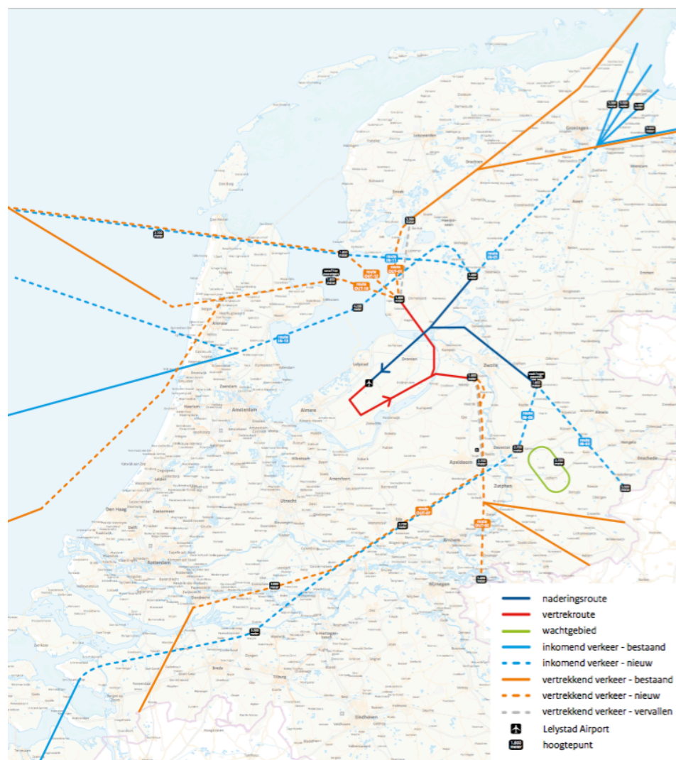
Figuur 2.2 Routestelsel voor uitgaand en inkomend verkeer bij starten en landen in zuidwestelijke richting; ongeveer 60% van de tijd. Zie bijlage 1 voor uitsneden met leesbare hoogteaanwijzingen. (versie 7 februari 2018).
